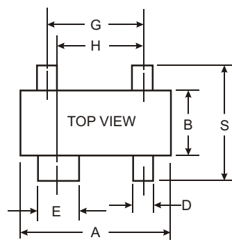
SOT-343 / SOT-143
