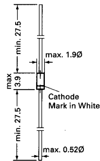
Glass case JEDEC DO-35
