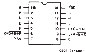
CD4025B
