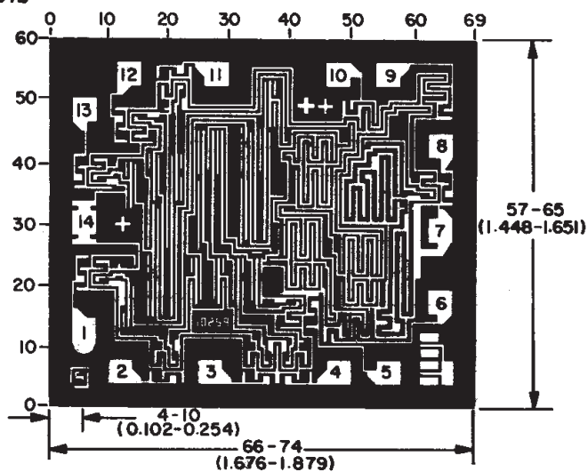
CD4025B
