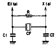
図2. 推奨発振回路
