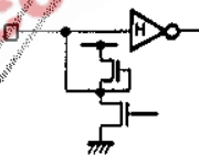
入出力共通ハイスレッシュヨルド入力プルアップ抵抗付 出力 (H, PU)
