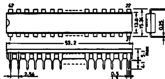
SANYO: DIP42
