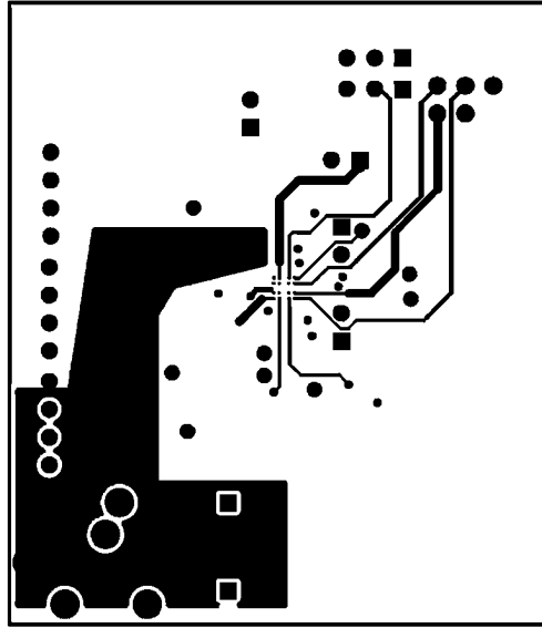
Layer 2
