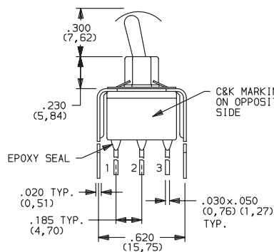
E101MD1_BE SPDT
