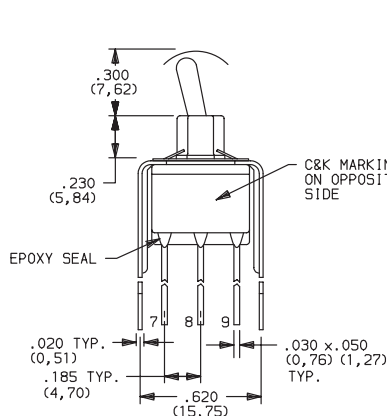
E301MD1_BE 3PDT
