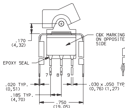
E301J1_BE2 3PDT
