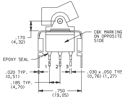
E101J1_BE2 SPDT
