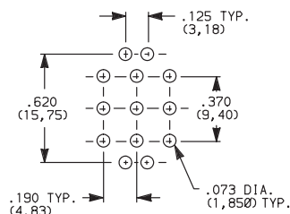
E301J1_BE2 3PDT
