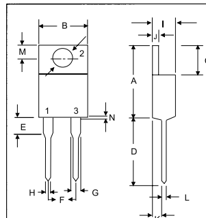
TO-220A
