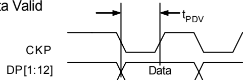
Data Valid
