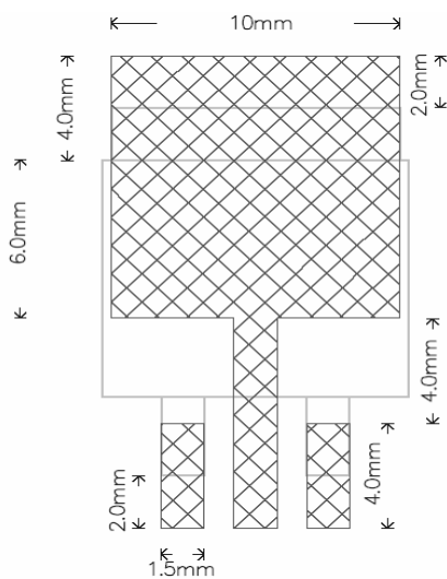
TO-263
