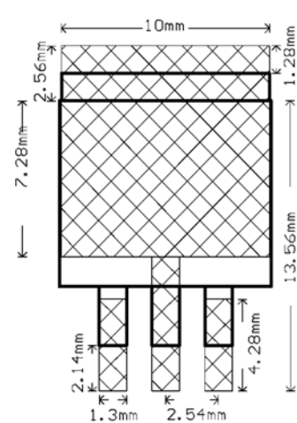
TO-263T
