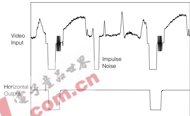
Fig. 16 Horizontal Output
