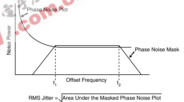
PHASE JITTER
