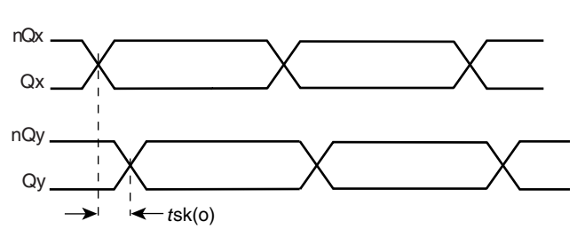
OUTPUT SKEW
