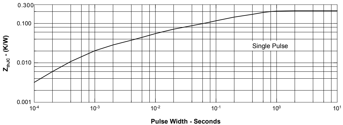
Fig. 10. Thermal Impedance
