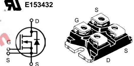
miniBLOC, SOT-227 B (IXFN)
