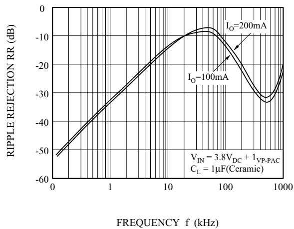
Fig. 8 PSRR
