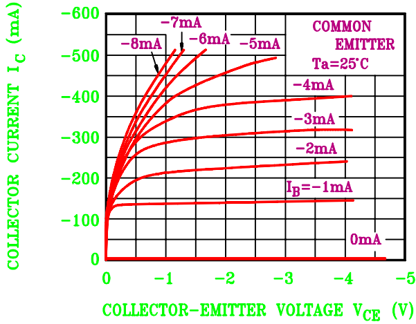
I_C - V_{CE}
