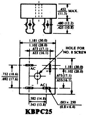
KBPC25
