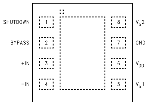
LLP Package
