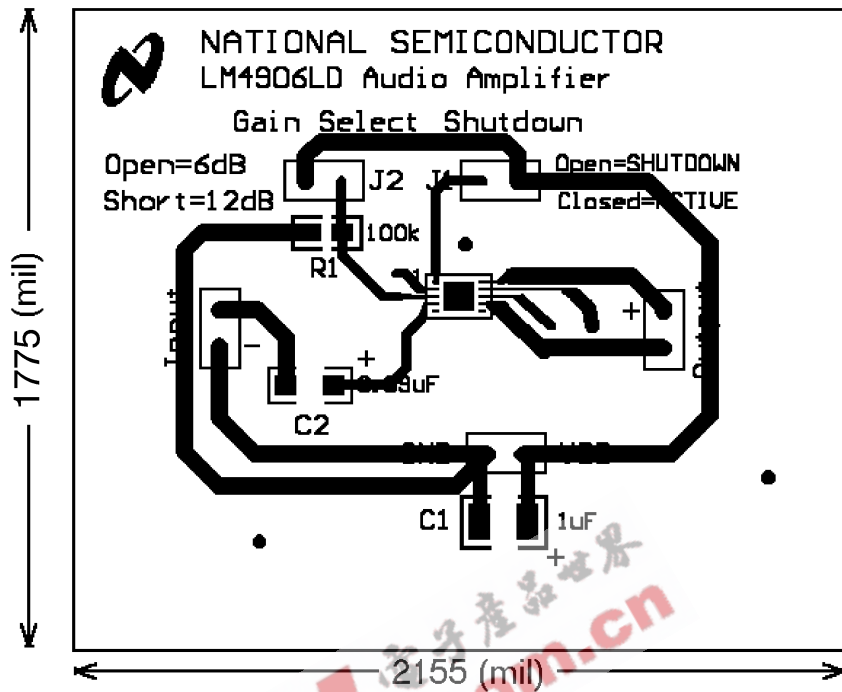
Top Layer
