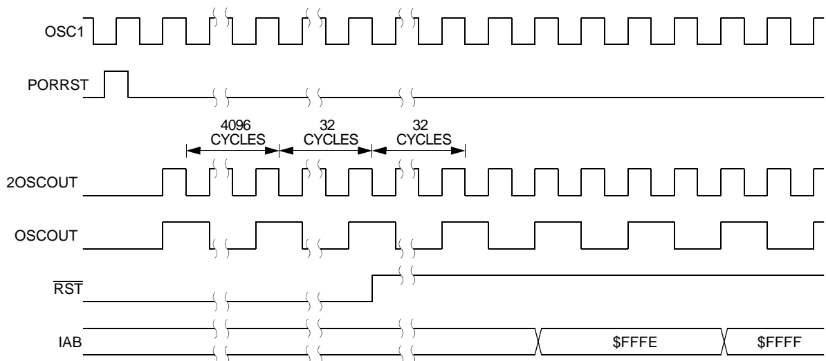
Figure 7-7. POR Recovery
