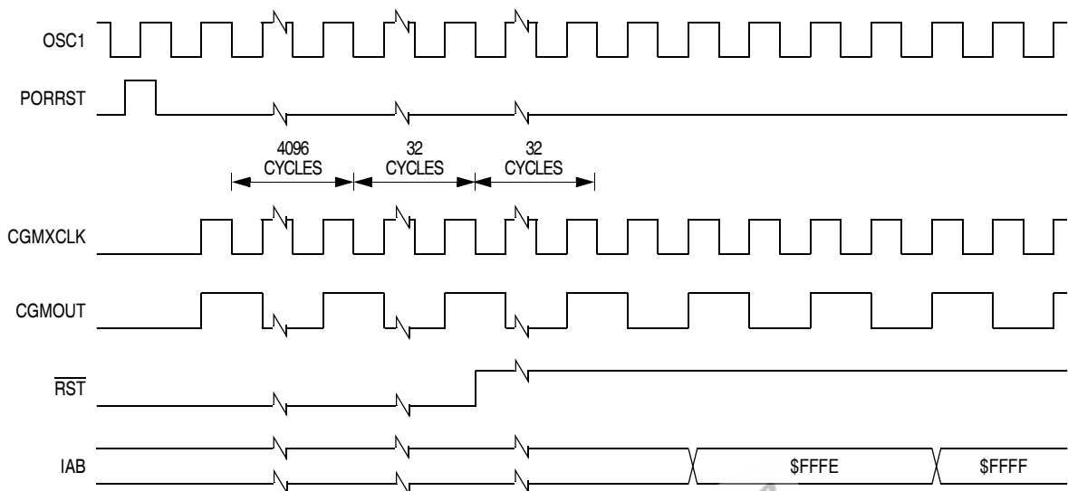
Figure 14-8. POR Recovery
