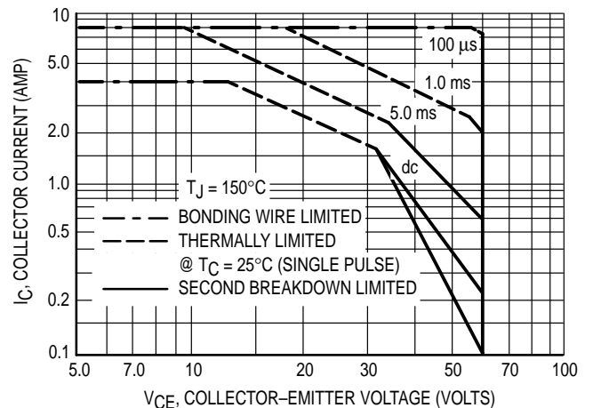
Figure 9. MJE800T
