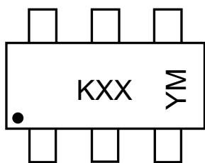
SOT-363
