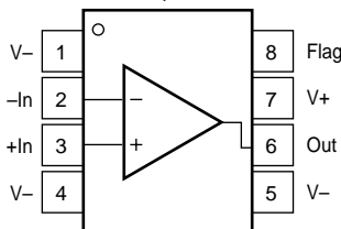
SO-8 (U)
