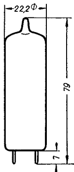
Kolbenabmessungen
