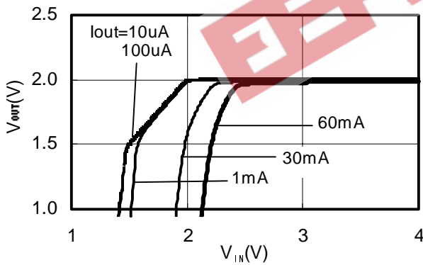
S-818A20A (Ta=25°C)
