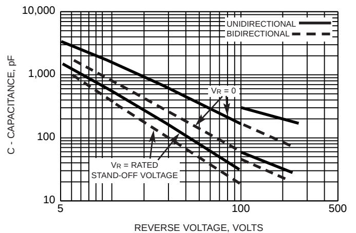
FIG. 6 - CAPACITANCE
