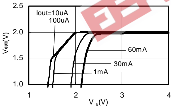
S-818A20A (Ta=25°C)
