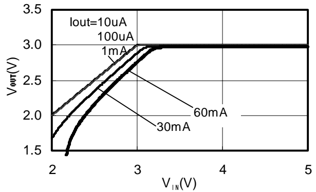
S-818A30A (Ta=25°C)
