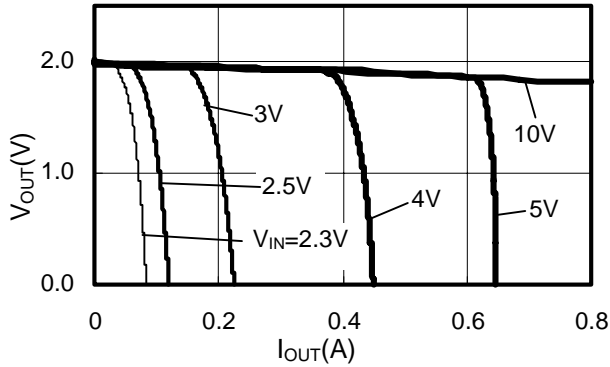
S-818A20A(Ta=25°C)
