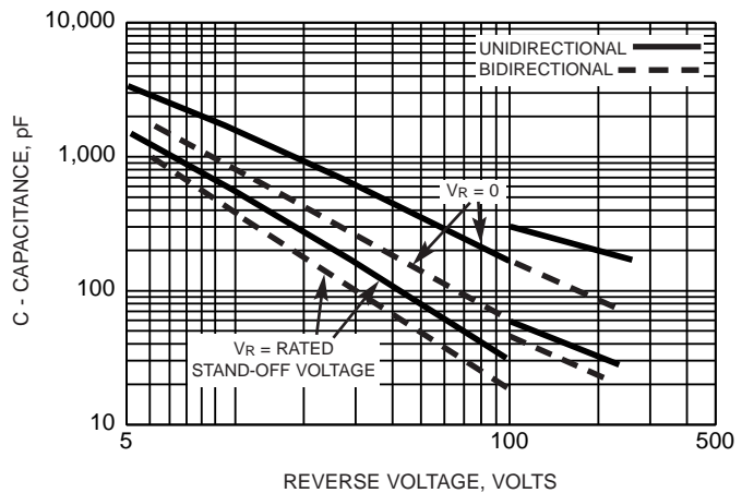
FIG. 6 - CAPACITANCE
