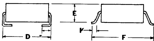
DO-214AA
