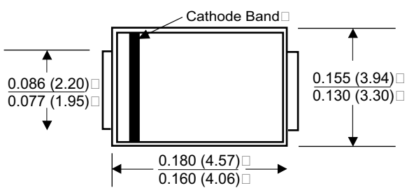
DO-214AA (SMB J-Bend)
