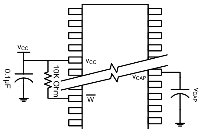
Figure 3. AutoStore Mode
