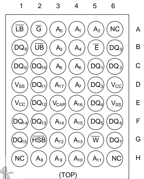
48-Ball FBGA
