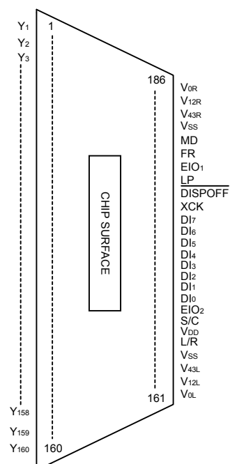
186 PIN TCP
