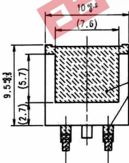
Fig. 1. P 矢視圖
