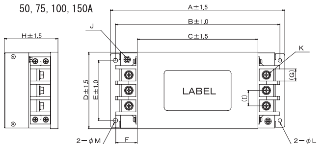
Dimensions
