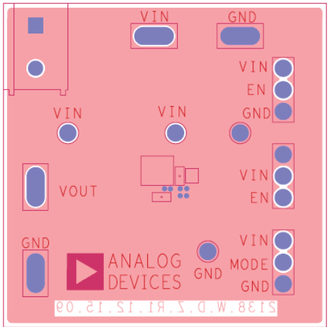
Figure 37. Bottom Layer
