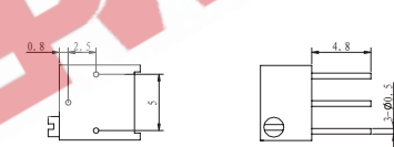
WIW1015-P
